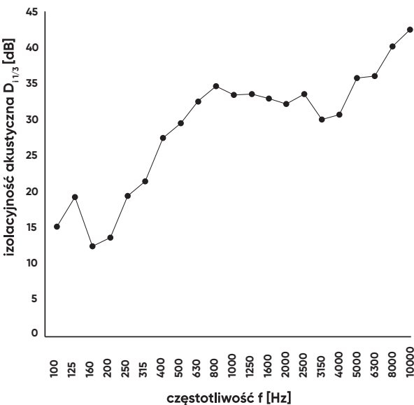
Ważony wskaźnik izolacyjności akustycznej
