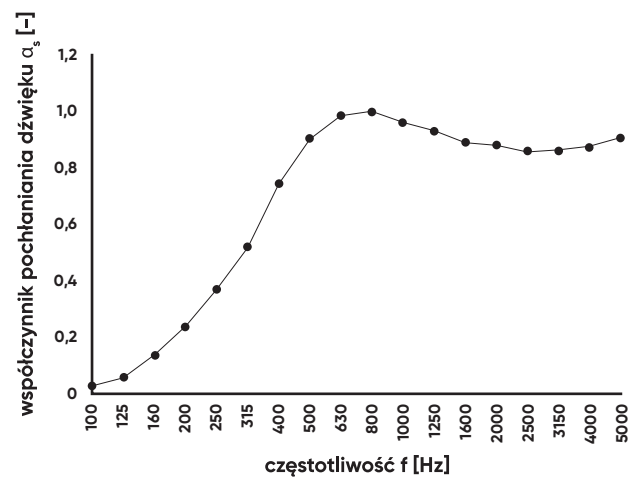
Pochłanianie paneli zewnętrznych Flathouse
